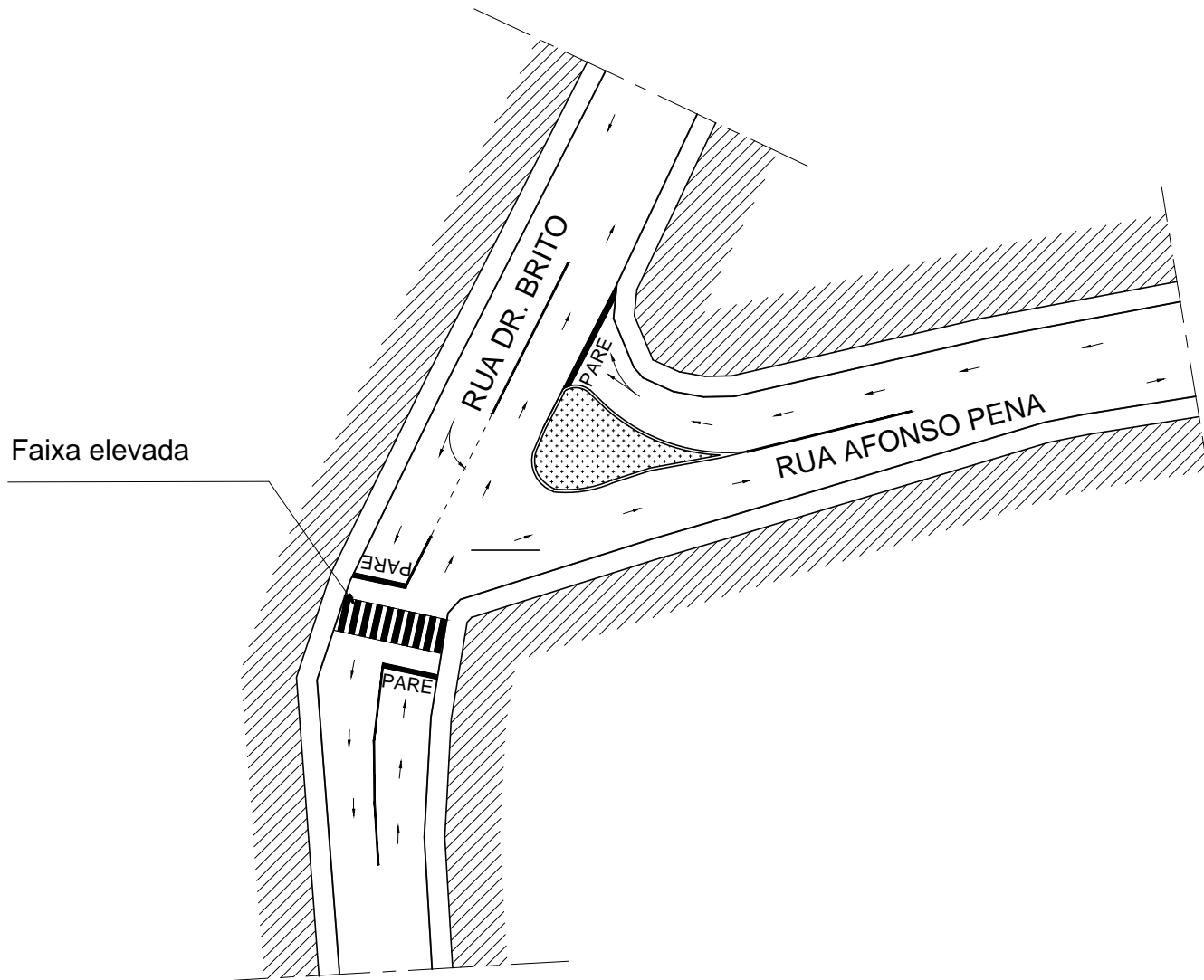
Interseção Rua Dr. Brito x Rua Afonso Pena ESC. 1:500
